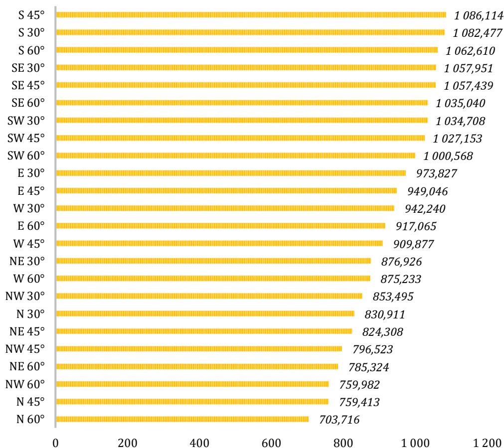
Wykres 33. Roczne wartości nasłonecznienia [kWh/m 2 ] dla określonej orientacji oraz pochylecia do płaszczyzny (dla stacji meteo we Wrocławiu)
